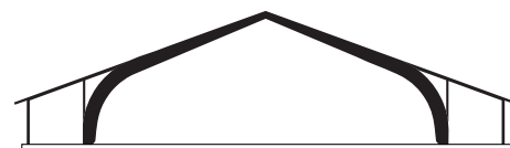
TRELEDSRAM MED KRÖKT RAMHÖRN Denna ramtyp används för spännvidder från ca 8 m till 40 m, och med taklutningar från 14° till ca 60°.
