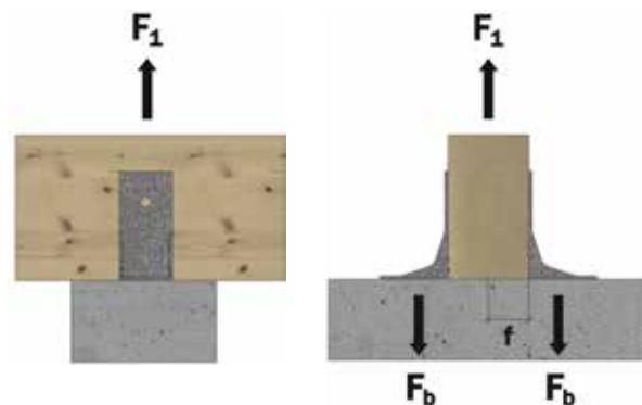
Søyle på betong, 2 vinkelbeslag pr. samling M12 bolt ned i betong
