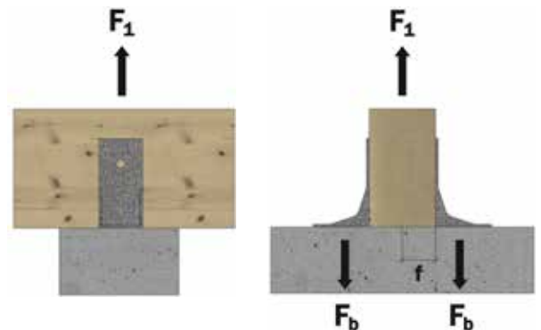
Søyle på betong, 2 vinkelbeslag pr. samling M12 bolt ned i betong
