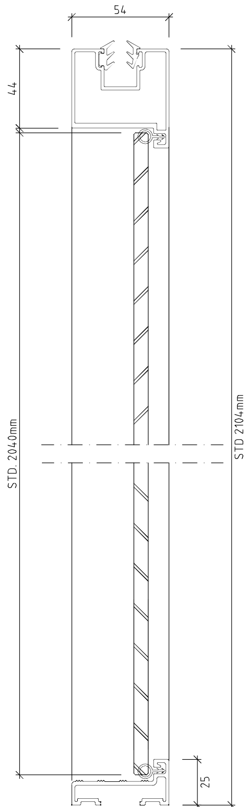
SEKTION A-A
